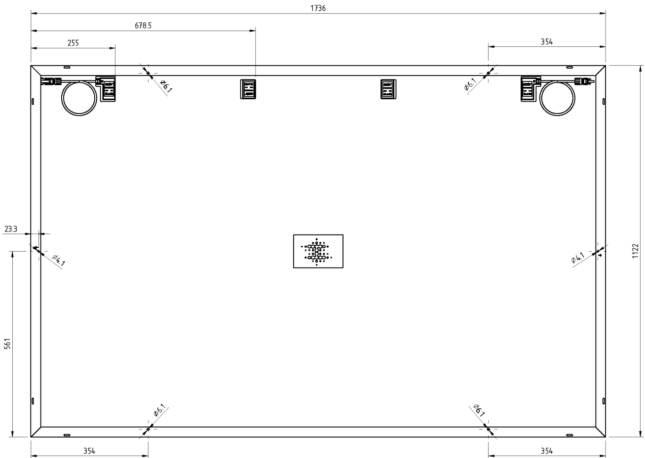
Abbildung 4: Anordnung Anschlussdosen
